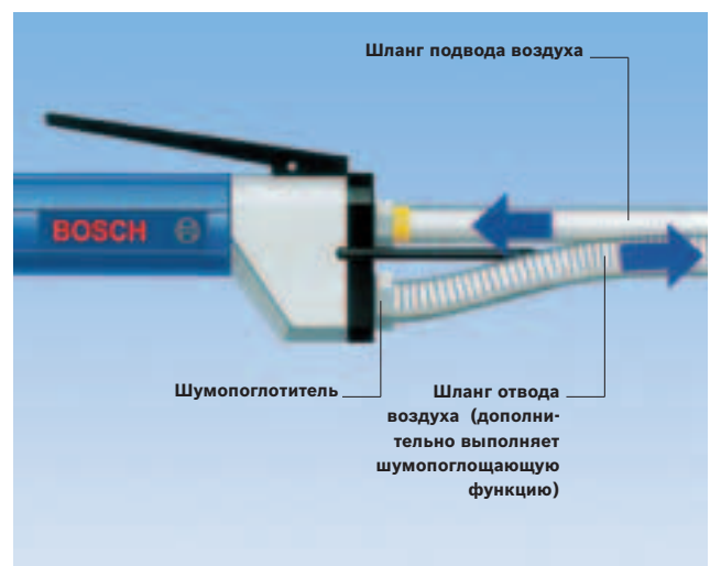
Рис. 7: Шланг отвода воздуха защищает пользователя, окружающую среду и обрабатываемую деталь
